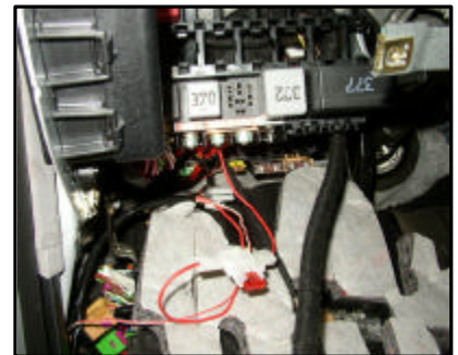
Anschluss des E-Satzes, Dauerstrom Modul
