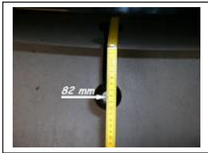
Abstand Mitte Kugelkopf zur Heckschürze 82mm
