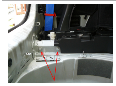
Stoßstange wie in der Anleitung beschrieben mit den Verstärkungsblechen befestigen: je 2 Schrauben am Heckblech (lange innen), 1 Mutter im Heckblech SW16) Innenansicht Befestigung Schrauben im Längsträger links SW16 ( Hier abgebildet ohne Verstärkungsblech! )
