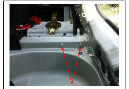
Innenansicht Befestigung Schrauben im Längsträger rechts SW16 ( Hier abgebildet ohne Verstärkungsblech! )
