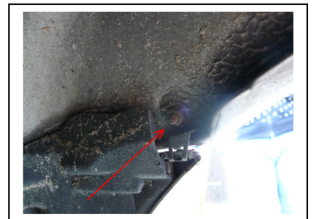
Demontage Stoßfänger links 1 Mutter (Halter für Clip)
